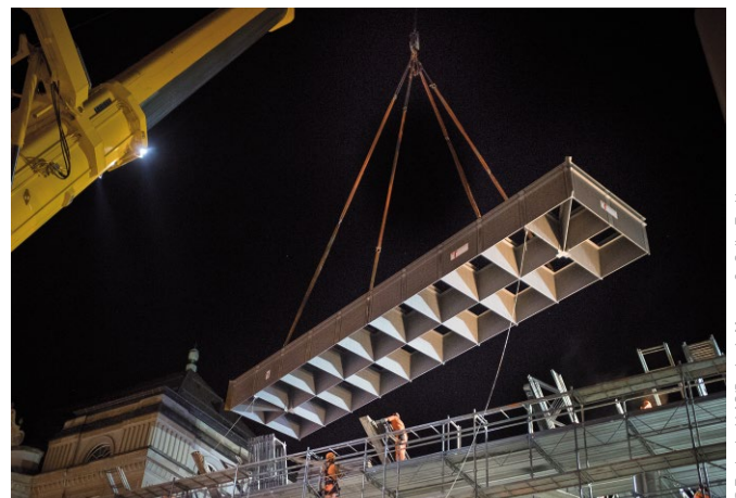
Bild 10 Nachtmontage Trägerrost-Element Night-time installation of a steel grid element
