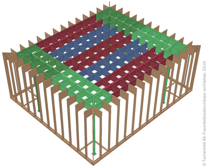
Bild 8 Montageablauf Installation process
