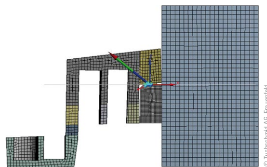
Bild 13 FE-Modell der Punkthalter FE model of the point fixings
