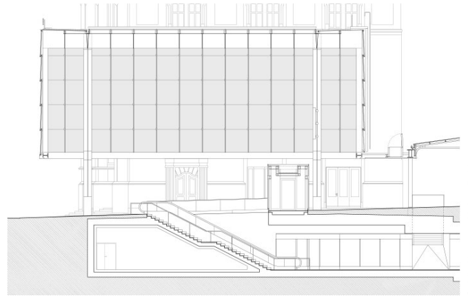
Bild 2 Längsschnitt Longitudinal section
