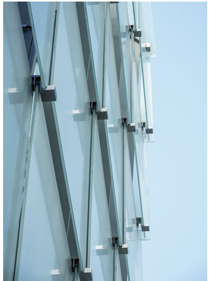
Bild 11 Detailansicht Glasfassade mit Punkthaltern Detail of the glass facade with point fixings
