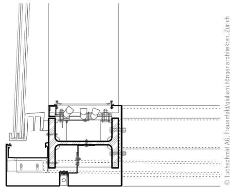
Bild 7 Untergurt HEM400 am Fuß der Stahlschwerter Bottom chord HEM400 at the bottom of the vertical steel elements supporting the facade
